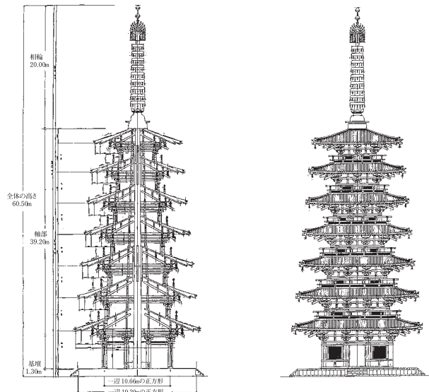
上野国国分寺七重塔復元設計図
